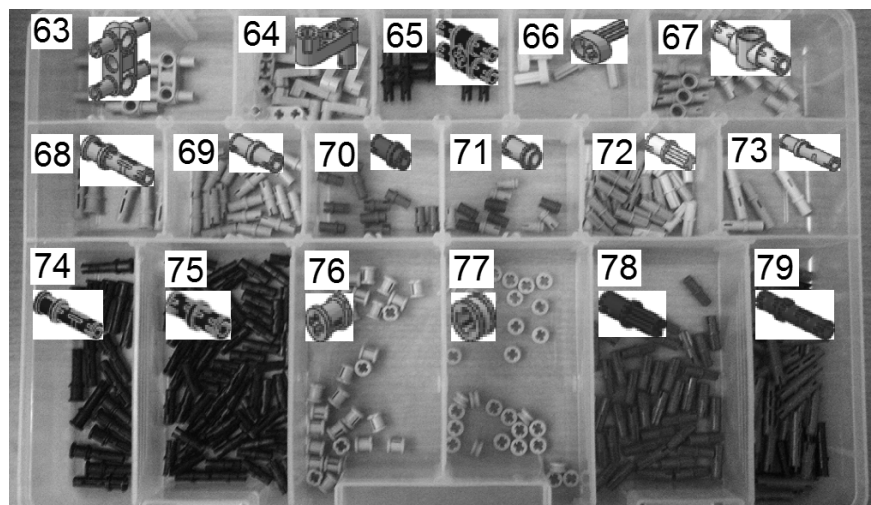
Rysunek 1-12 Kolekcja łączników sworzni i tulei Technic
